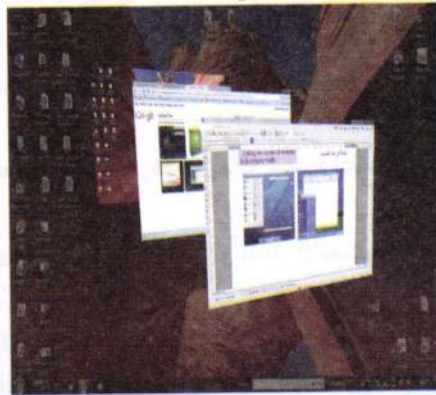
ويندوز 7 Windows 7
